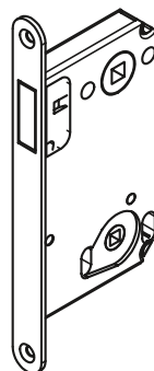
magnetický zámek WC
