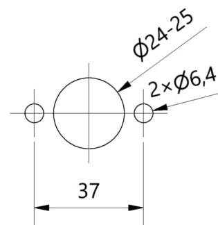
vrtání otvorů pro MG rozety
