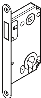
magnetický zámek cylindrický
