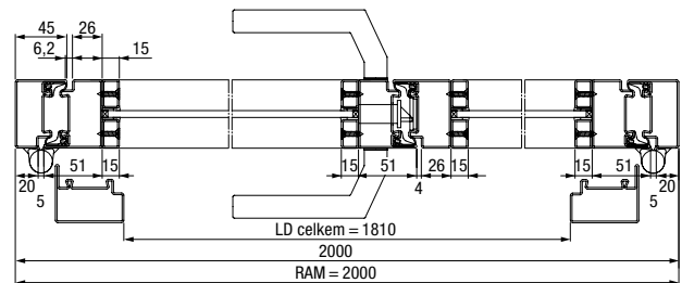
Vodorovný řez dvoukřídlými ocelovými loftovými dveřmi
