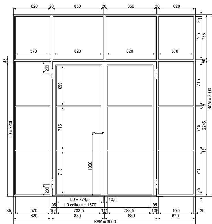
Dvoukřídle ocelové loftové dveře s bočními díly a horním světlíkem
