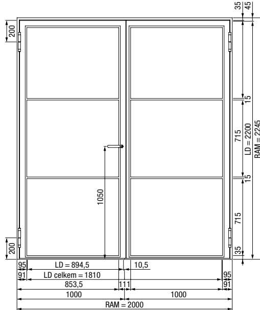
Dvoukřídlé ocelové loftové dveře
