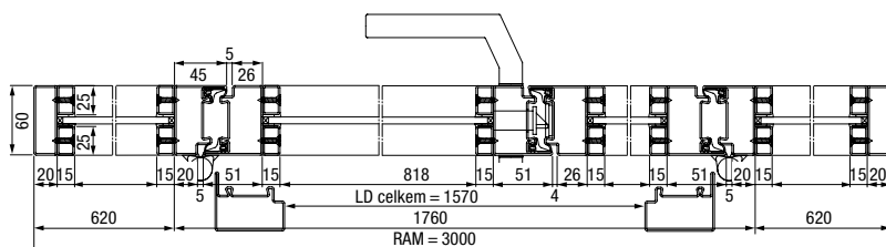
Vodorovný řez dvoukřídlymi ocelovými loftovými dveřmi s bočními díly a horním světlíkem
