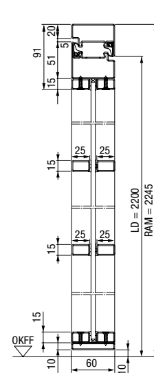
Svislý řez jednokřídlými ocelovými loftovými dveřmi
