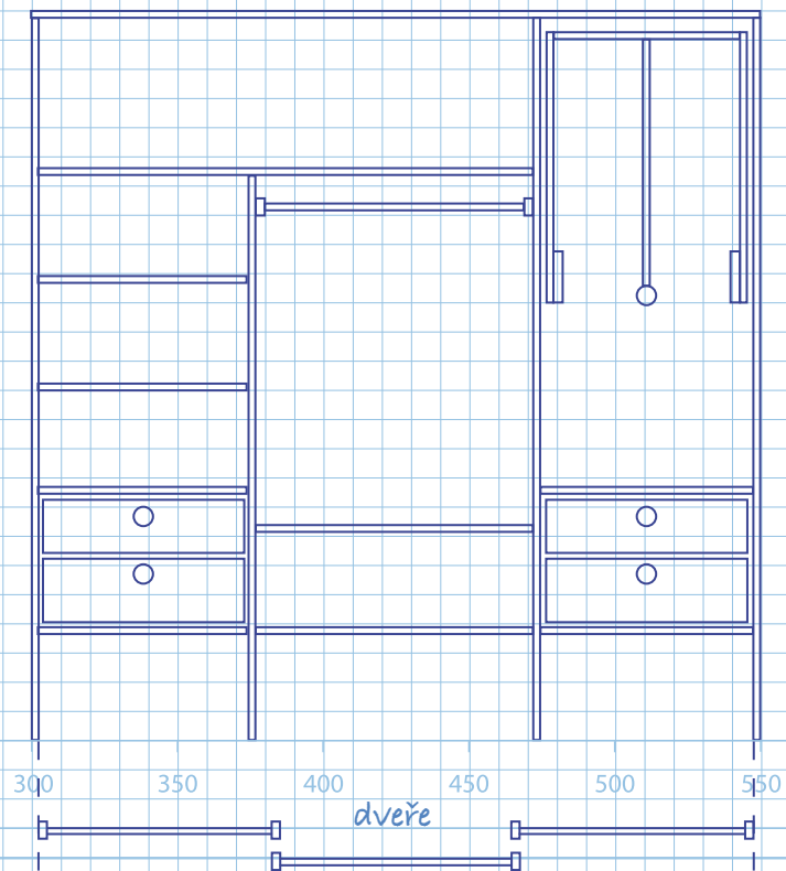
Návrh skříně pro dvě osoby
