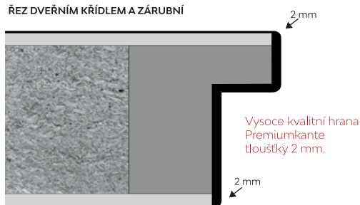
DVEŘNÍ KŘÍDLO S HRANOU PREMIUMKANTE (PK)
